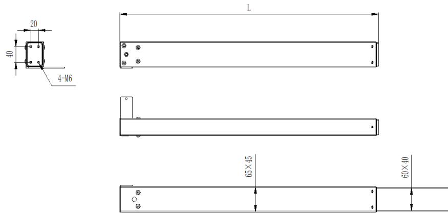
左腿外形图
